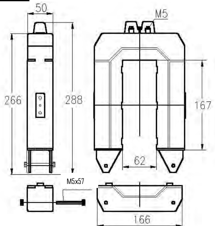
Габаритный чертеж
